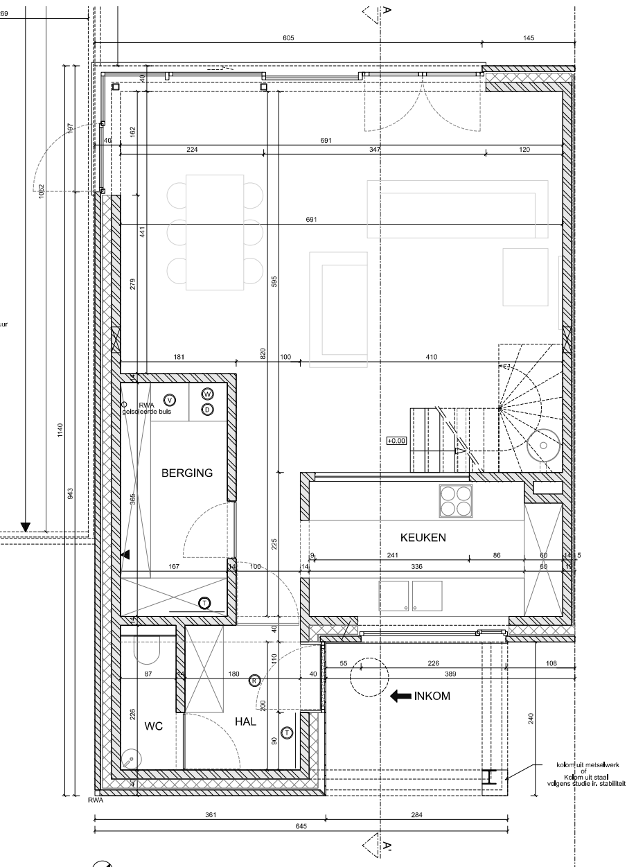
GELUIKVLOERS schaal: 1/50
